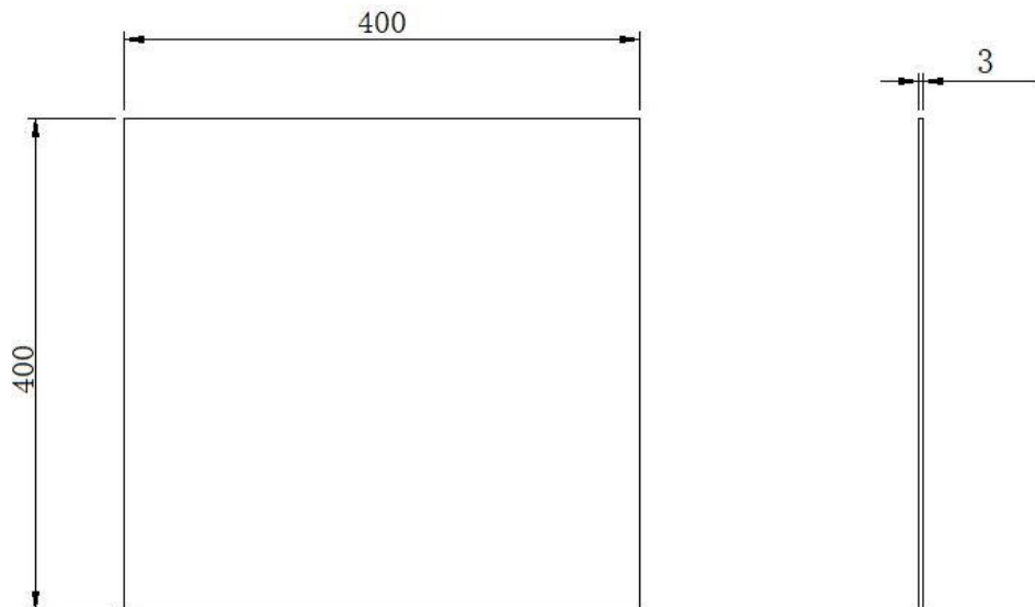
(图4) 铝散热板尺寸图
