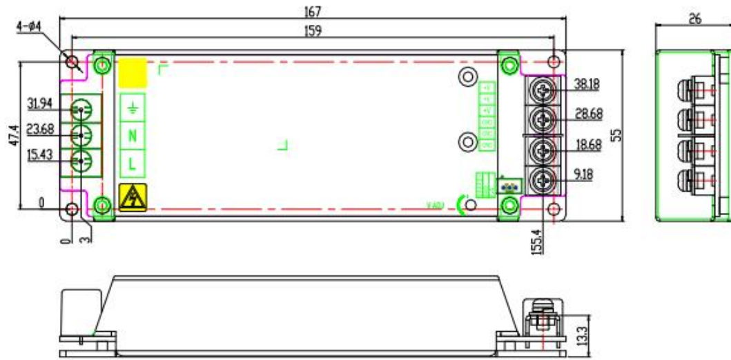
外形尺寸及安装孔——端子坐标图
