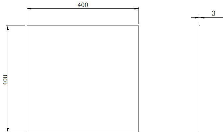
(图 4) 铝散热板尺寸
