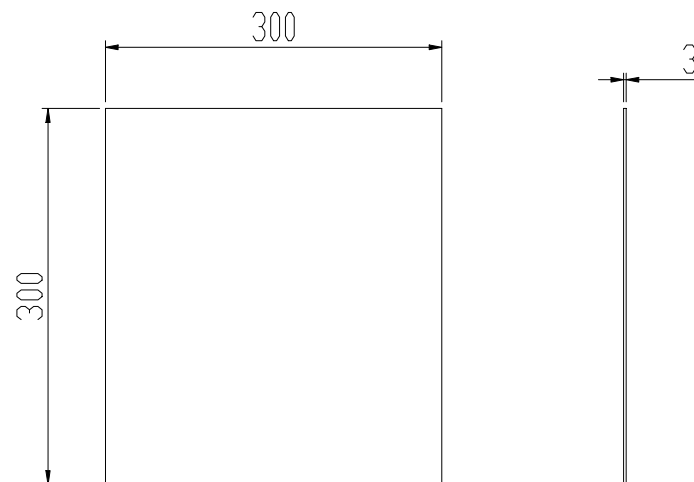
图4 铝散热板尺寸图
