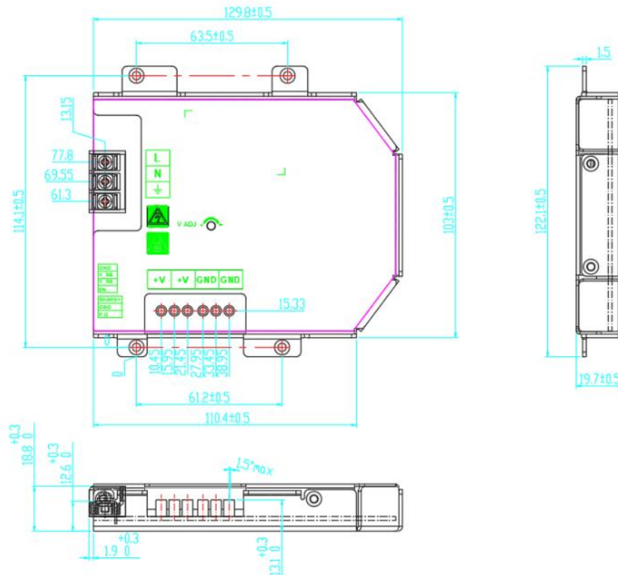
外形尺寸及安装孔——端子坐标图
