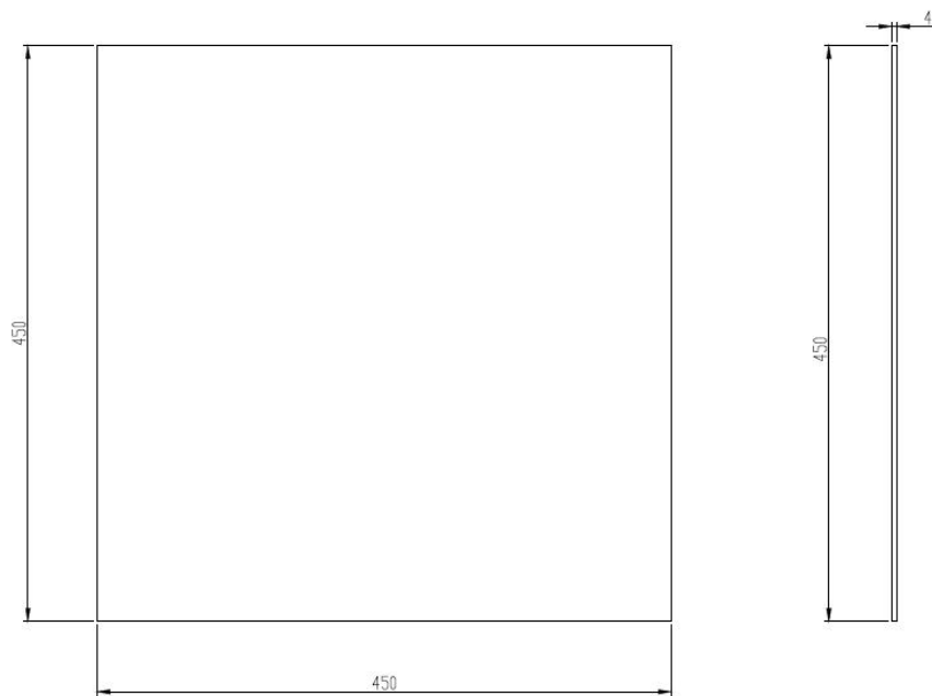
图4 铝散热板尺寸图
