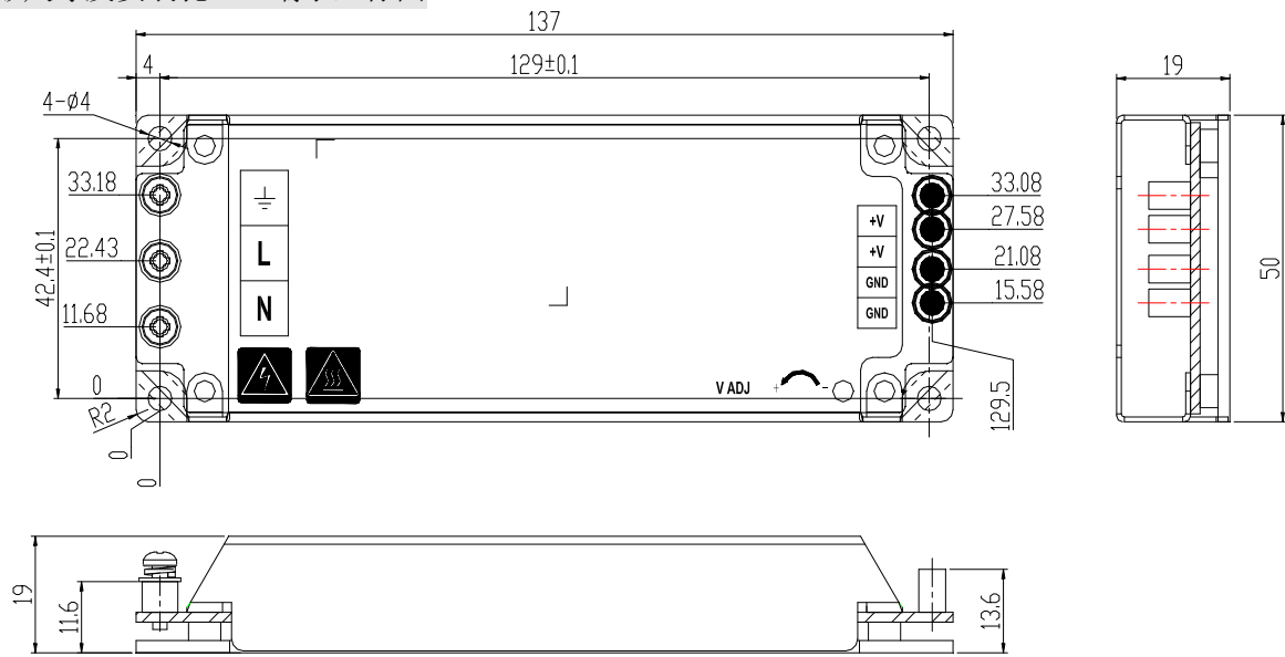
外形尺寸及安装孔——端子坐标图
