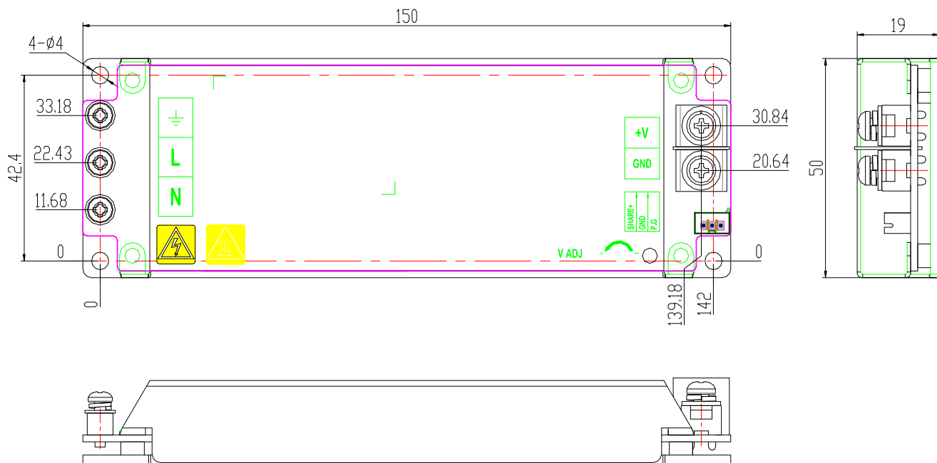
外形尺寸及安装孔——端子坐标图
