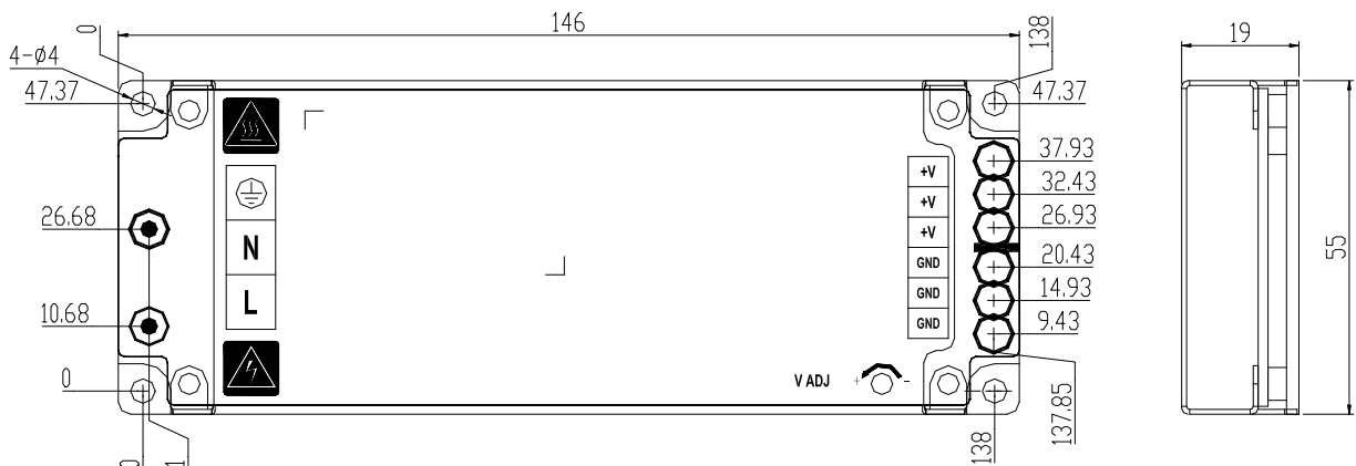
外形尺寸及安装孔——端子坐标图
