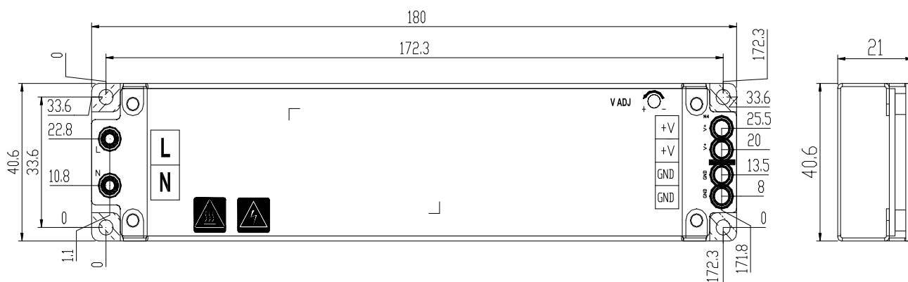
外形尺寸及安装孔——端子坐标图
